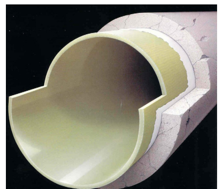
Nach dem Aushärten entsteht ein komplett neues Rohr im alten Rohr.
