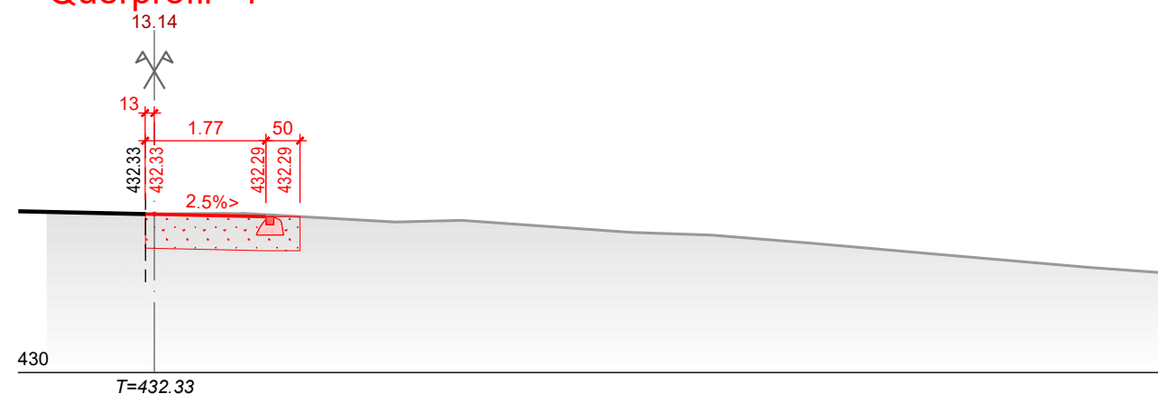
Querprofil 1
