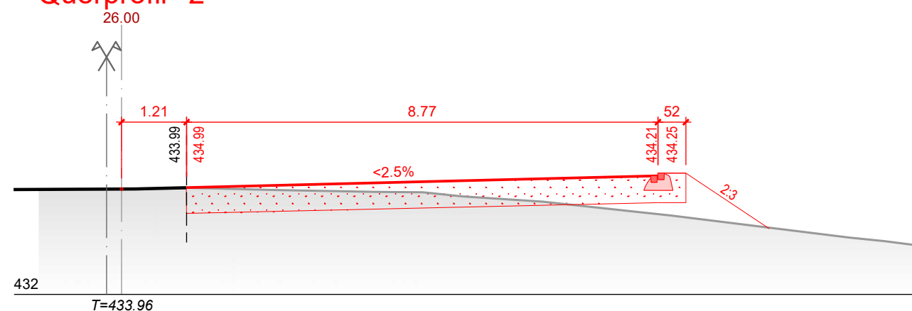
Querprofil 2
