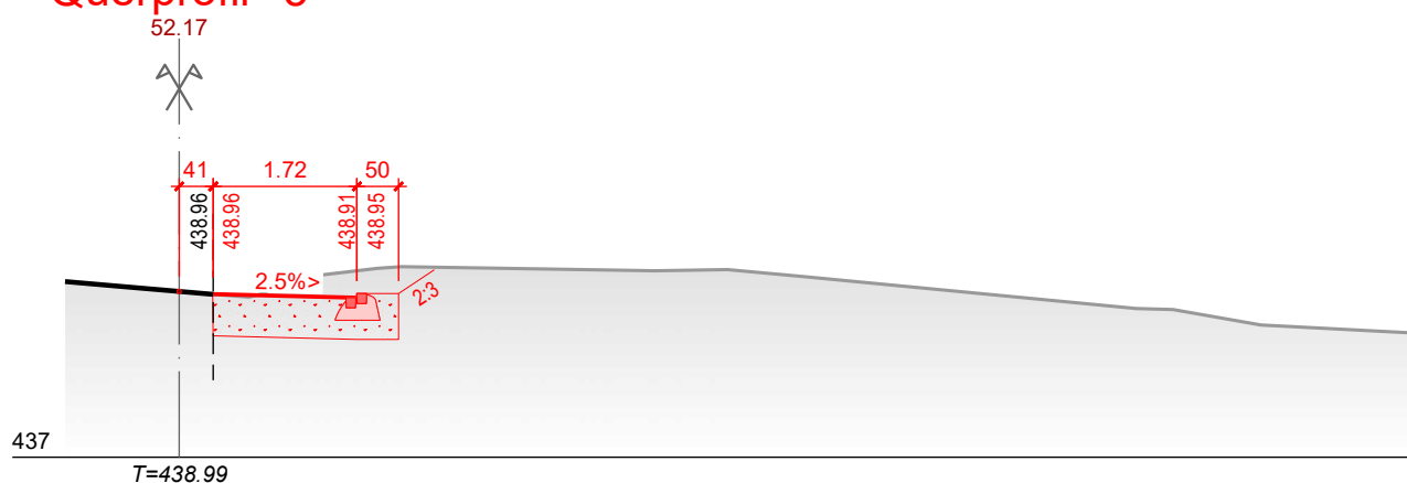
Querprofil 5
