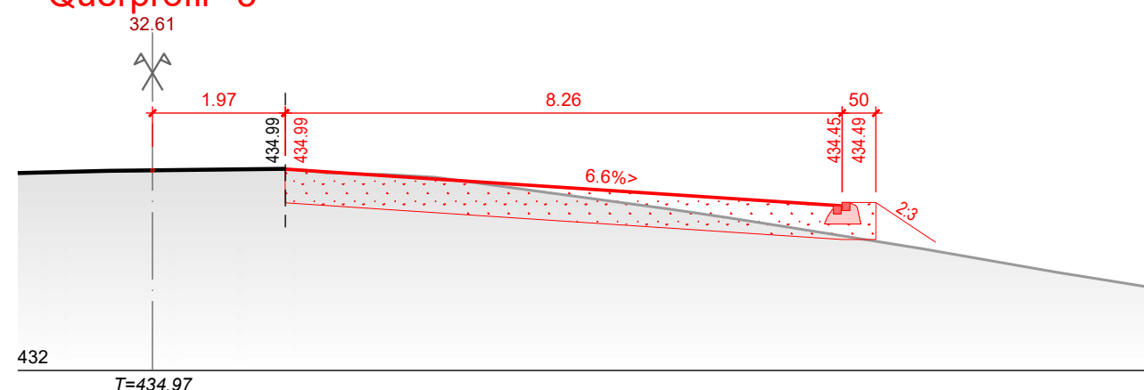
Querprofil 3
