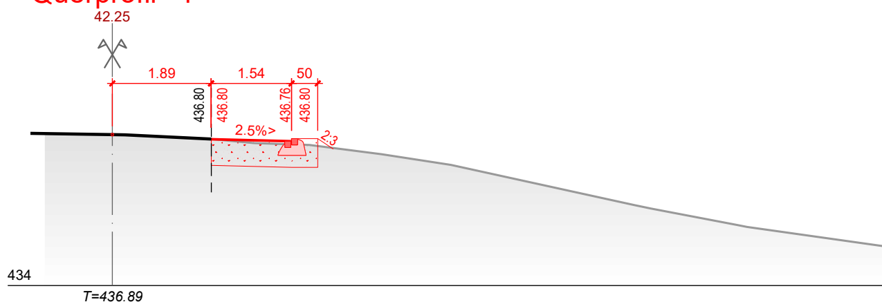
Querprofil 4
