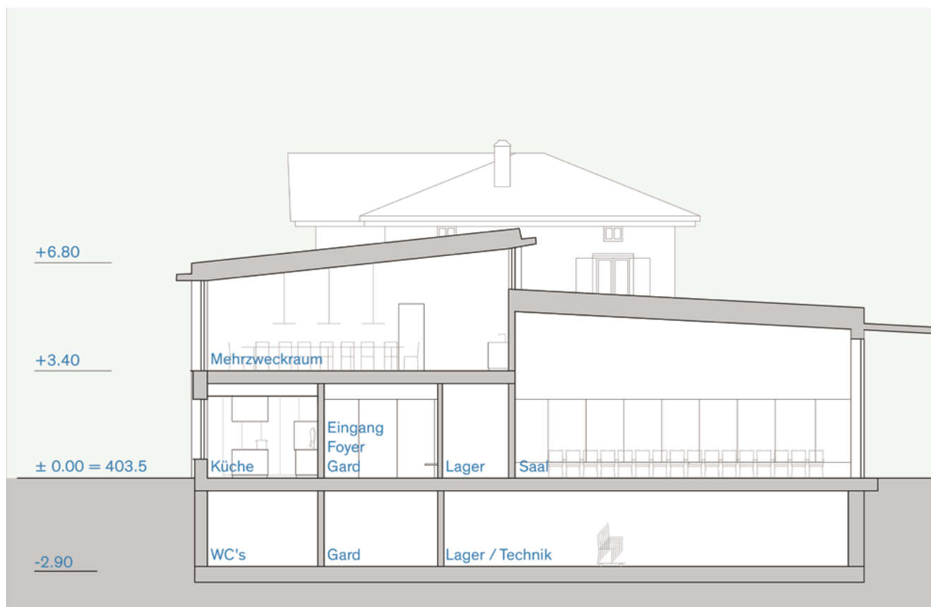
Querschnitt
