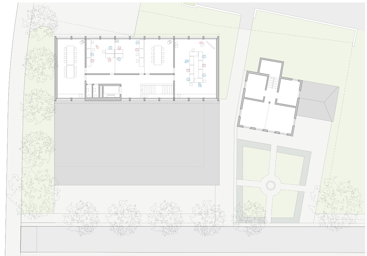
Obergeschoss
