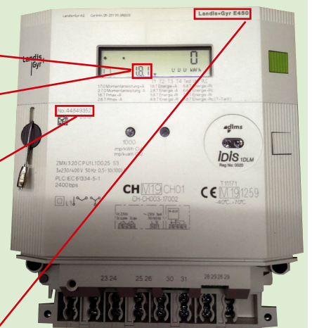
Smartmeter Landis+Gyr E450
