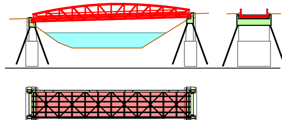
4. Brücke fertigstellen
