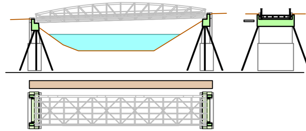
3. Instandsetzung Brücke gemäss Vorschlag Unternehmer
